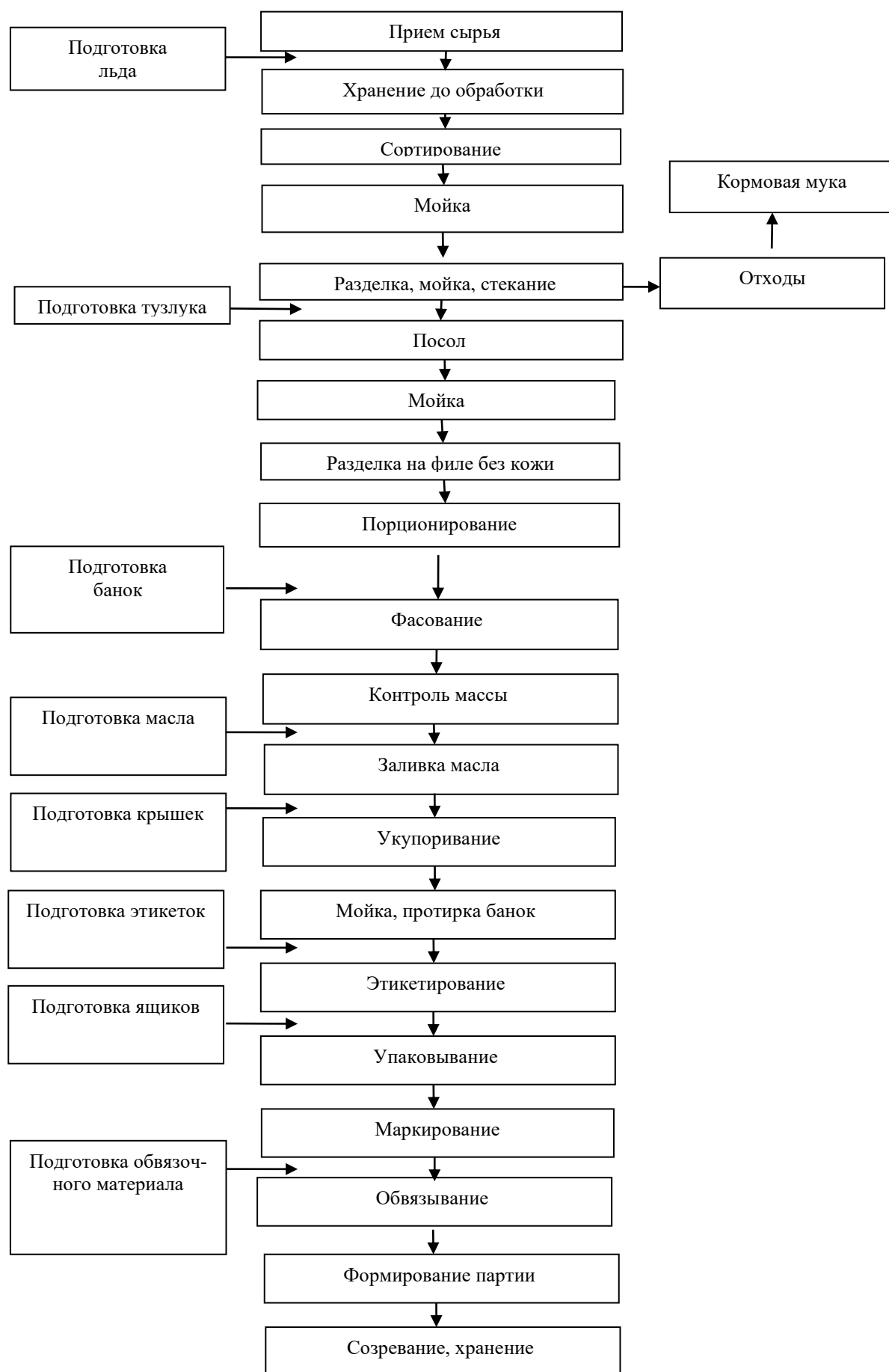
Рис. 3.2 – Технологическая схема производства пресервов «Горбуша филе-ломтики в масле»
