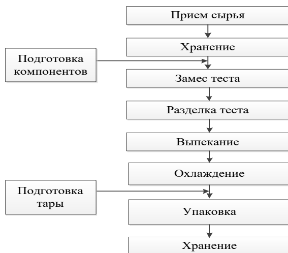
Рисунок 3.2 – Технологическая схема производства сдобных изделий
