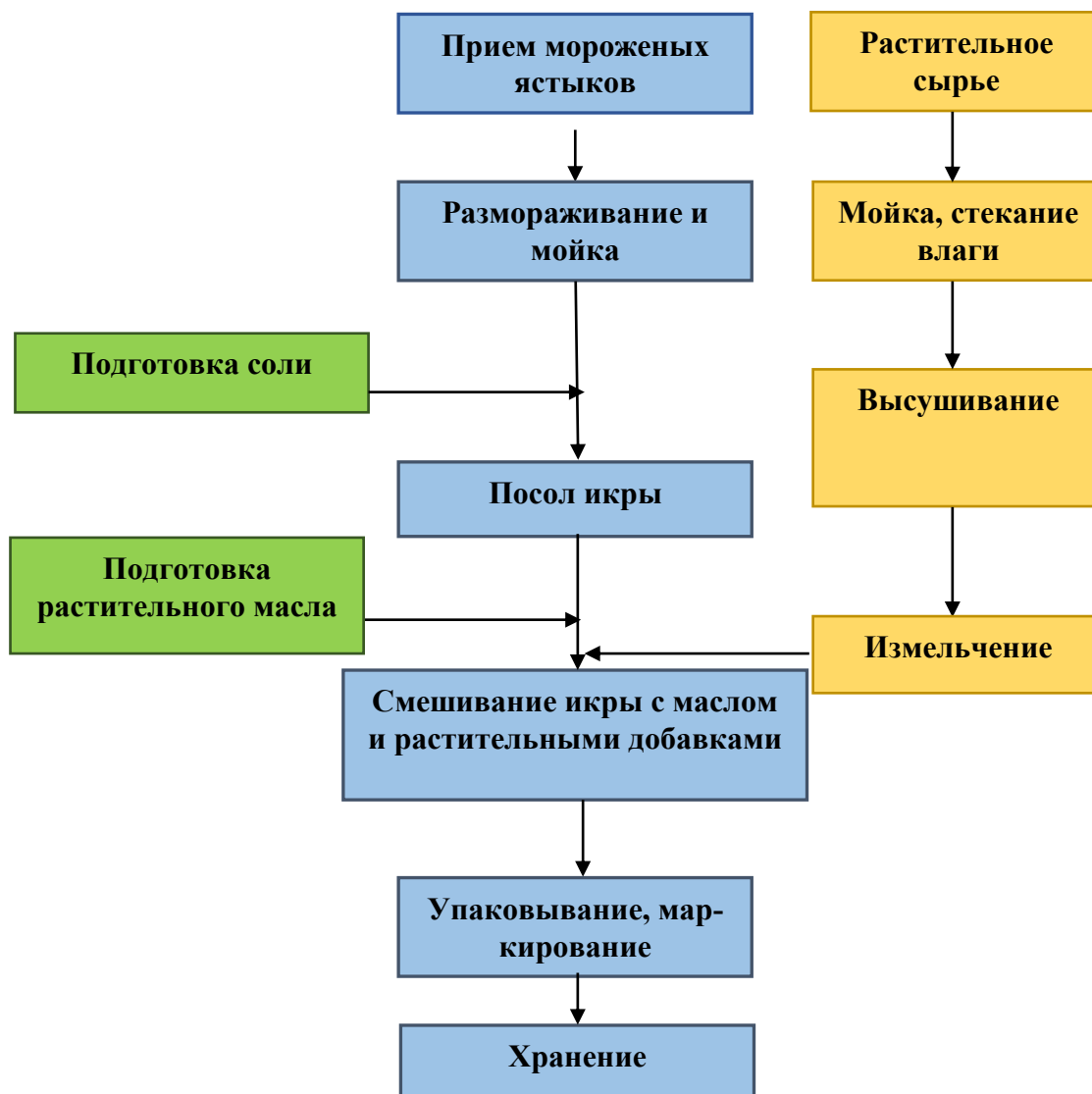
Рисунок 3.2 – Технологическая схема производства икры сельди соленой ястычной с растительными добавками
