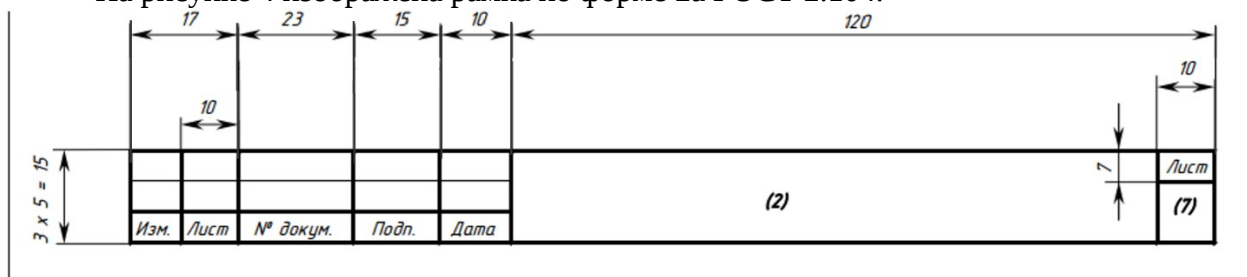
Рисунок 4 – Форма 2а основной надписи по ГОСТ 2.104 ЕСКД
