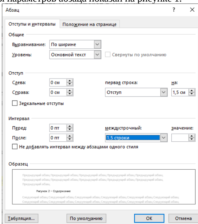
Рисунок 1 – Параметры абзаца
